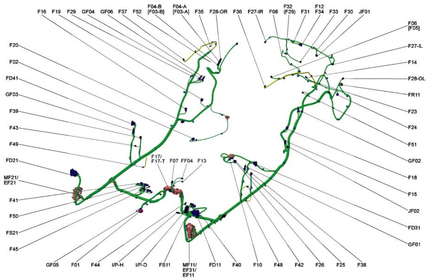
底板线束(1)
